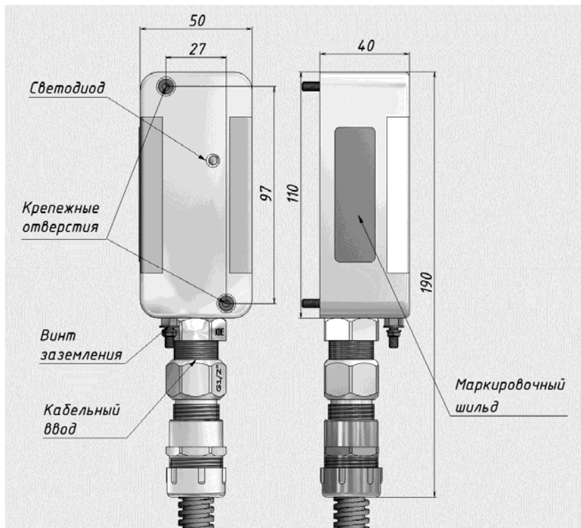
Рис.1 Габаритно-установочные размеры изделия
